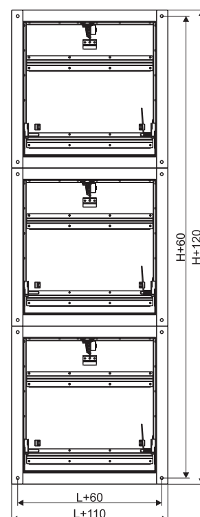
3и - три кассеты по H (3 привода)
