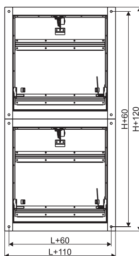
2и - две кассеты по H (2 привода)
