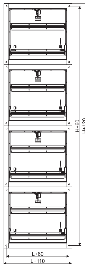
5и - четыре кассеты по H (4 привода)
