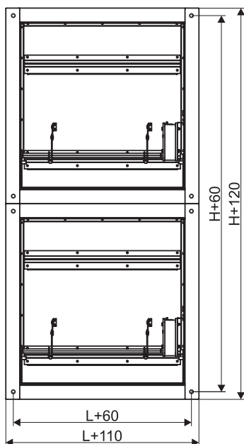
4и - две кассеты по H (2 привода)
