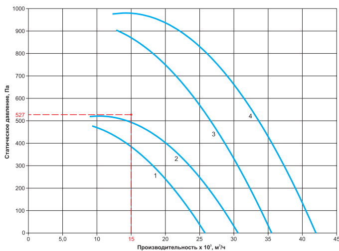
Аэродинамические характеристики вентиляторов РОКС-ВКРС-9,0-ДУ, РОКС-ВКРФ-9,0-ДУ
