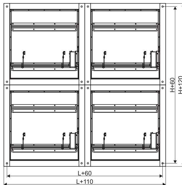
5и - две кассеты по L, две кассеты по H (4 привода)
