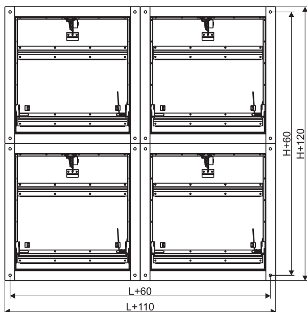
6и - две кассеты по L, две кассеты по H (4 привода)
