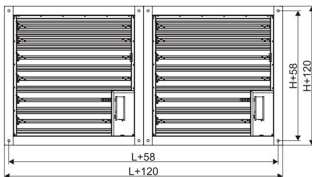
2и - две кассеты по L (2 привода)
