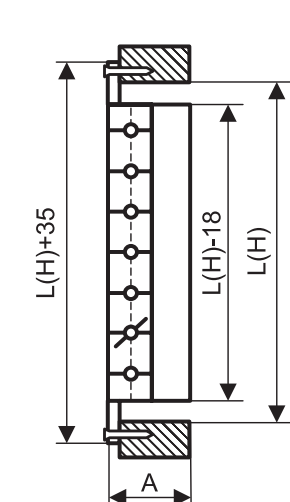
Монтаж с помощью самонарезающих винтов
